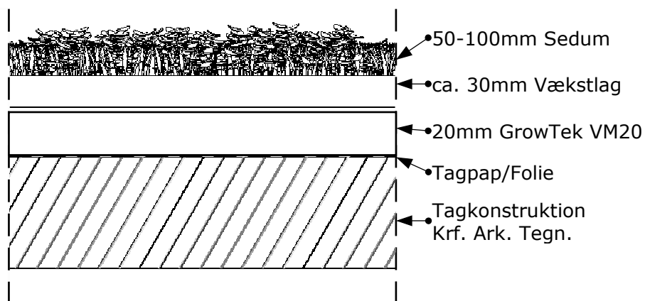
Principsnit GrowTek VM20 sedum tag
