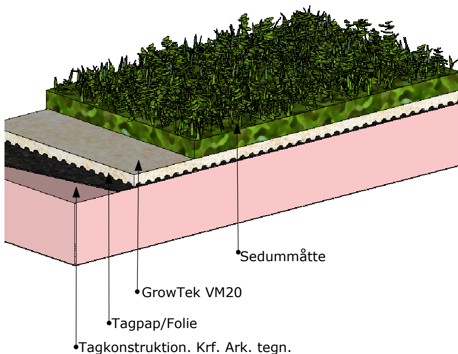
Principopbygning GrowTek VM20 sedum tag
